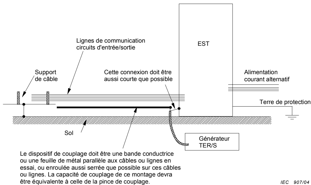
Figure 13 – Exemple d'essai sur site sur les accès de communication et d'entrée/sortie sans la pince de couplage capacitive
