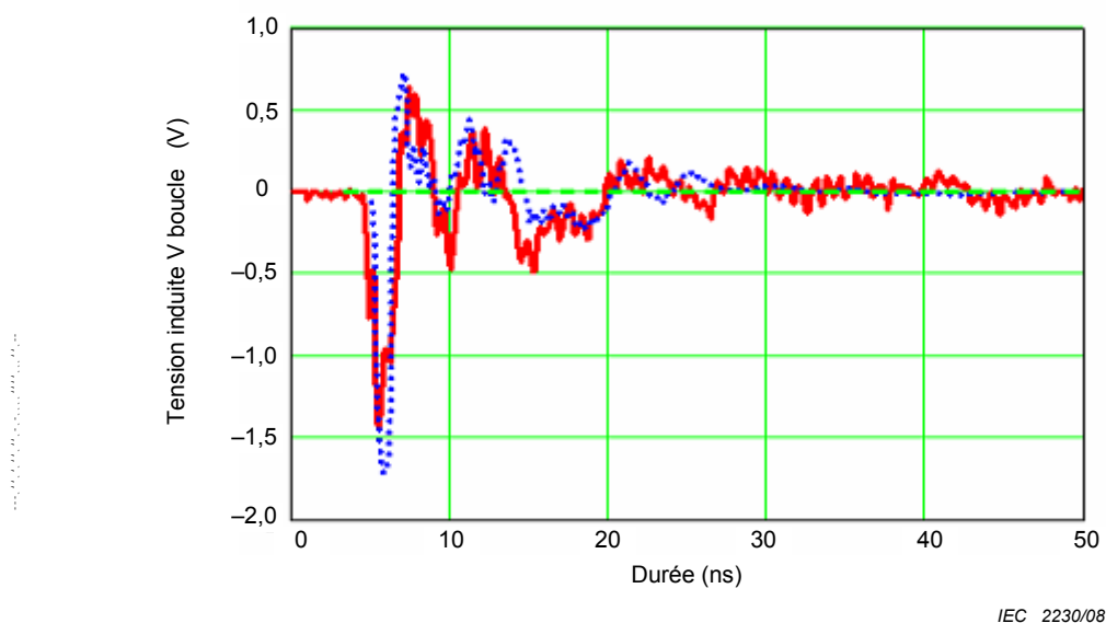
Figure D.6 – Comparaison entre la chute de tension mesurée (trait plein) et la valeur calculée numériquement (trait pointillé) sur la boucle pour une distance de 45 cm
