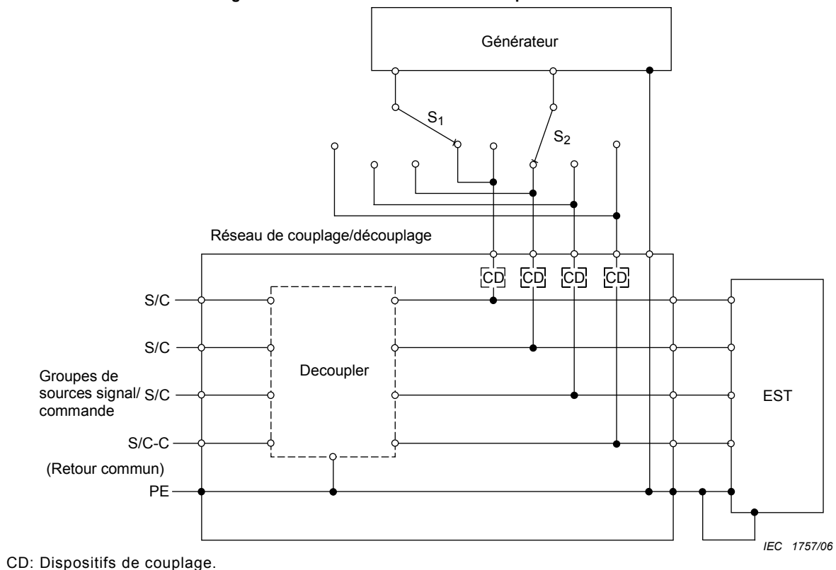
Figure 12b – Installation d'essai avec connexions de terre spécifiques
