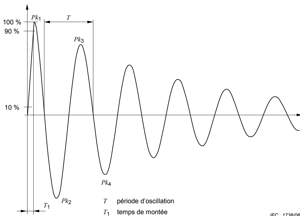
Figure 1 – Forme d'onde de l'onde sinusoïdale amortie (tension en circuit ouvert)
