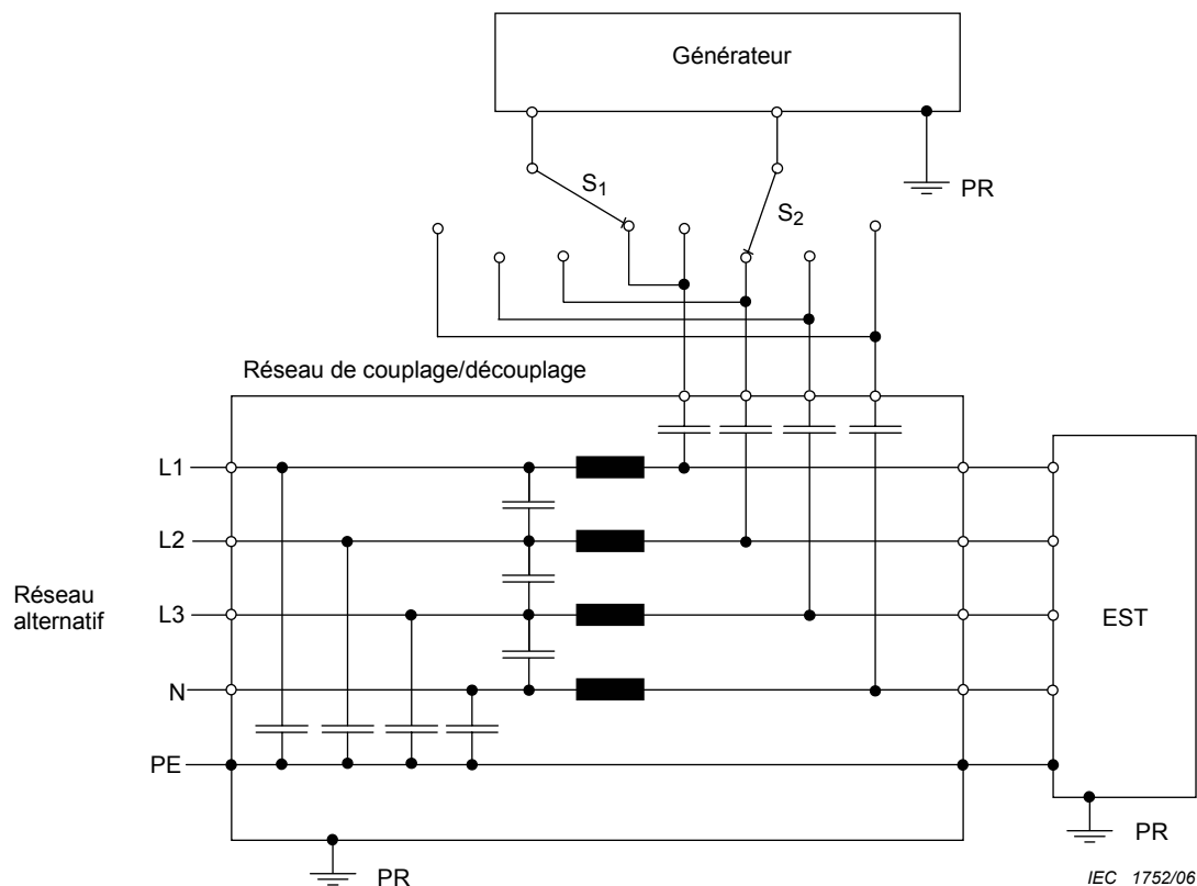
Figure 10a – Installation d'essai avec plan de référence
