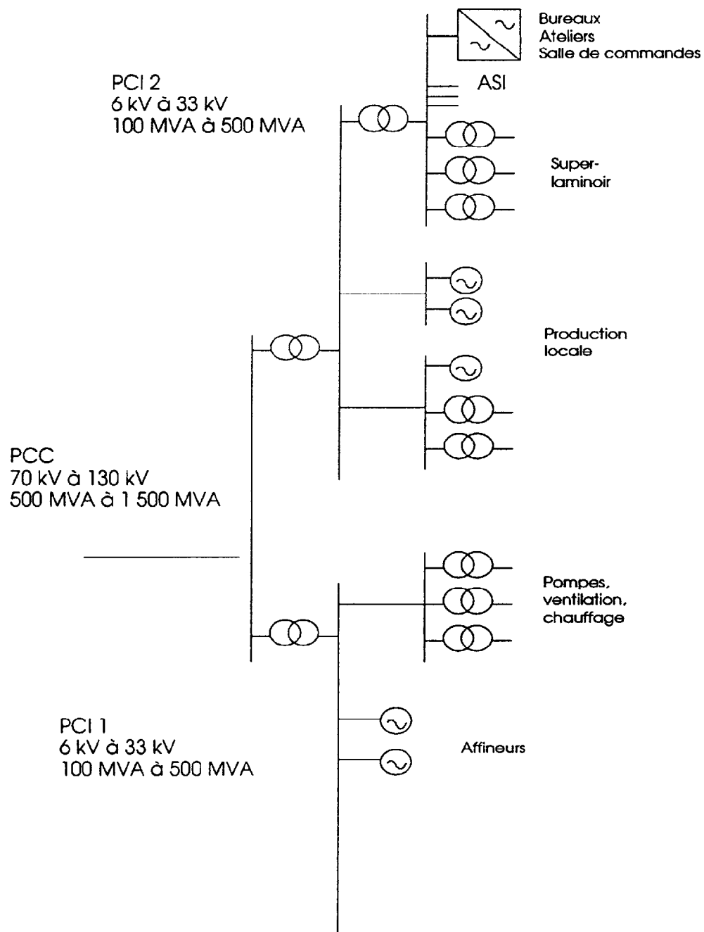
Figure A.2 – Exemple de distribution de puissance dans l'industrie papetière
