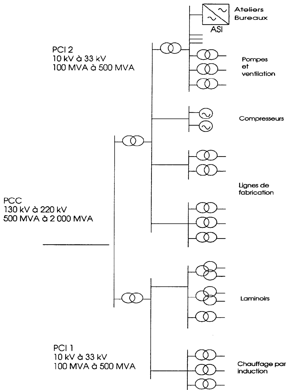
Figure A.1 – Exemple de distribution de puissance dans une industrie comprenant des laminaires
