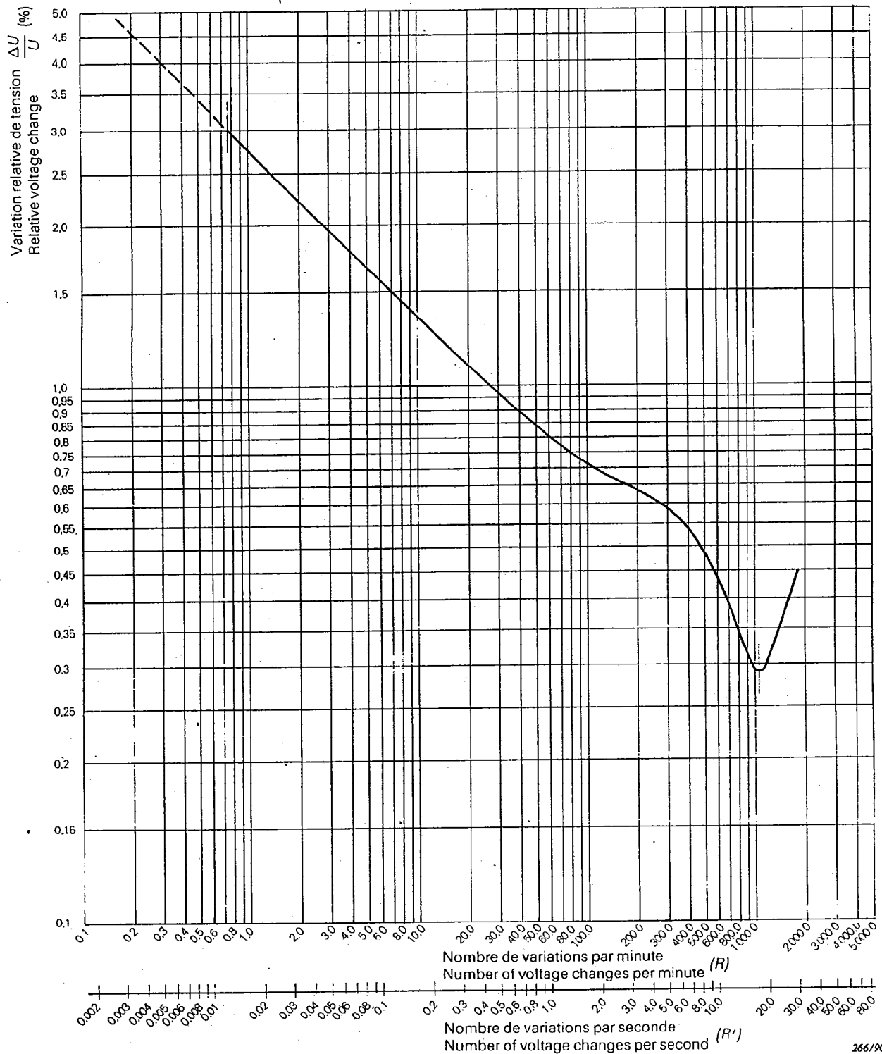
Figure 1 - Variations de tension en créneau et flicker: Amplitude des variations maximales admissibles de tension \Delta U/U (%) en fonction du nombre de variations de tension par seconde ou par minute
